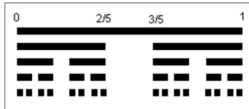
C_5 : dimension \approx 0.7565
